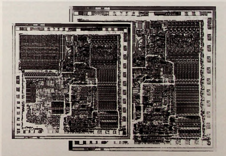
Bild 2.1: Mikroskopaufnahmen moderner hochintegrierter Schaltungen. Auf einer Kristallfläche von ca. 5×5 mm sind 29 000 Transistoren untergebracht
