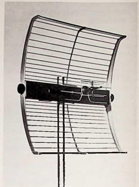
Bild 8: CLOU 45, eine komplett vormontierte UHF-Hochleistungsantenne kurzer Bau-länge für reflexionsreiche Empfangslagen (fuba-Presebild)
