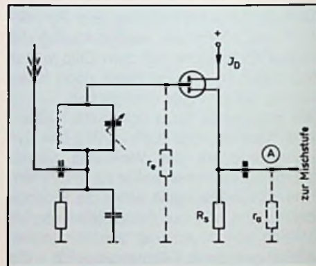
Bild 2: Direkt an den Vorkreis angeschalteter FET in Drainschaltung zur optimalen Anpassung an die Mischstufe
