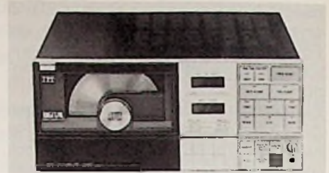
Bild 4: Digital Audio Player Typ HiFi 9015 von ITT
