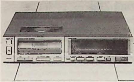
Bild 6: Der schon bekannte Schublader CD-73 von MARANTZ
