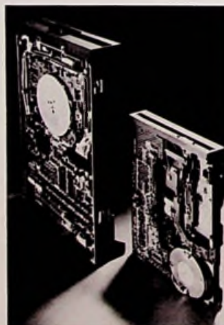
Bild 1: Flache Floppy-Disk-Laufwerke (links Typ 6105, rechts 6138) (Feltron-Pressbild)
