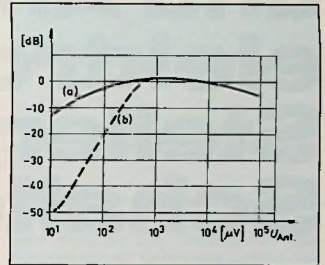
Bild 6: NF-Ausgangsspannung in Abhängigkeit von der Antennen-Eingangsspannung bei einer AM-Empfängerschaltung (a) ohne (b) mit FET-Zwischenstufe nach Bild 2 (über DIN-Kunstantenne; 1 MHz; m = 30\% )
