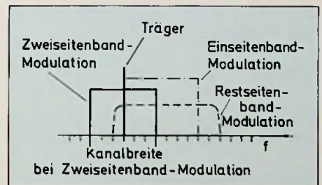
Bild 2: „Aufmodulieren“ von Informationen auf eine „Trägerwelle“ ( f = \text{Frequenz} )
