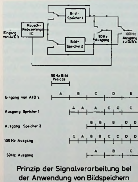
Bild 1: Prinzip der Signalverarbeitung bei der Anwendung von Bildspeichern.
