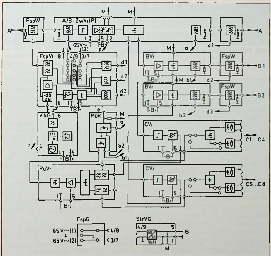
Bild 5: Blockschaltbild eines BK-Verstärkerpunktes
