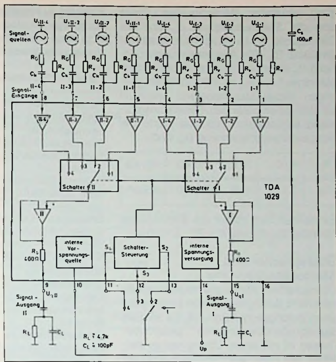
Bild 20: Blockschaltung des Signalquellenschalters TDA 1029 mit externer Beschaltung
