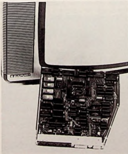
Bild 1: Diskret aufgebauter Btx-Decoder (Blaupunkt-Pressbild)
