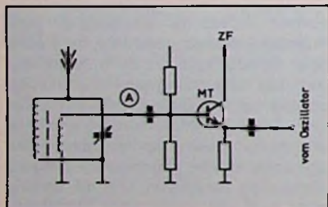
Bild 1: Die in AM-Eingangsschaltung übliche induktive Ankopplung des Eingangskreises an den Mischtransistor MT
