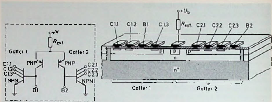
Bild 2.9: Logikschaltung in I 2 L-Technologie
