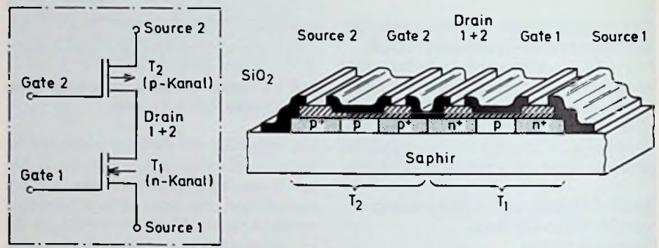
Bild 2.10: CMOS-Inverter in SOS-Technologie
